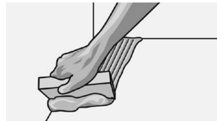
Рис. 107. Клей наносится на основание специальным гребенчатым шпателем только под приклеиваемый ряд досок. После укладки полного ряда необходимо зафиксировать и прижать доски к фанерному основанию с помощью паркетных гвоздей или специальных шпилек, применяя пневмоинструмент.
