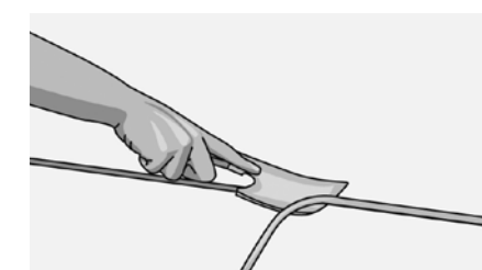
Рис. 37. Второй срез делается после того, как сварочный шнур окончательно остыл.
