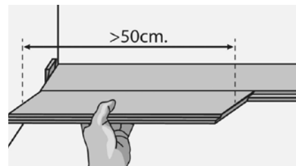
Рис. 108. Сборка очередного ряда начинается с остатка доски предыдущего ряда, при условии, что длина оставшегося фрагмента не менее 50 см. Монтаж нового ряда следует начинать с соединения торцевых кромок доски, и дальнейшей стыковкой по длинной стороне. Необходимо контролировать, чтобы все расстояния между торцами досок соседних рядов было не менее 50 см, это придаст паркету необходимую прочность.
